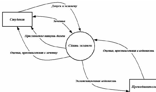
Рисунок 1. – DFD-диаграмма процесса «Сдать экзамен».
