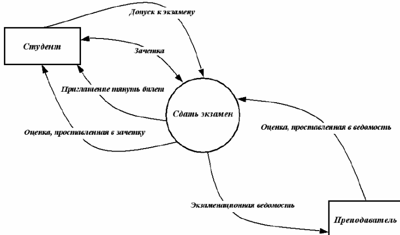
Рисунок 1. – DFD-диаграмма процесса «Сдать экзамен».
